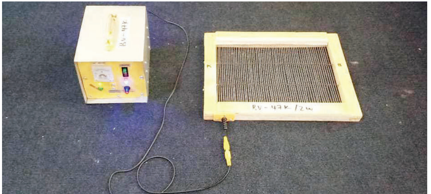
Kifaa cha kunasa sumu ya nyuki kinachofaa na kuendana na mazingira ya Tanzania. PICHA: CHRISTINA MWAKANGALE
