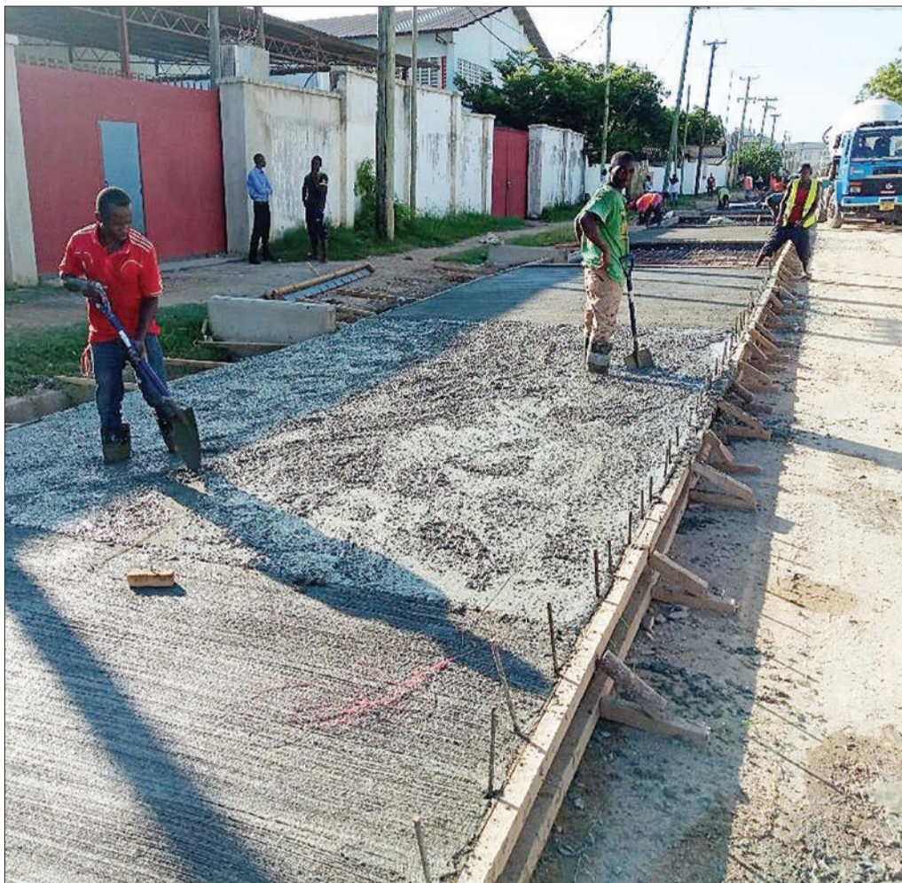
Mafundi wakimwaga zege kwenye barabara inayotoka ITV kuelekea nyumba za maafisa wa serikali. PICHA: JOSEPH MWENDAPOLE
